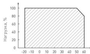
Рис. 3. Максимальная допустимая нагрузка, % от мощности источника.
